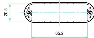
A-A (1:1.5)
